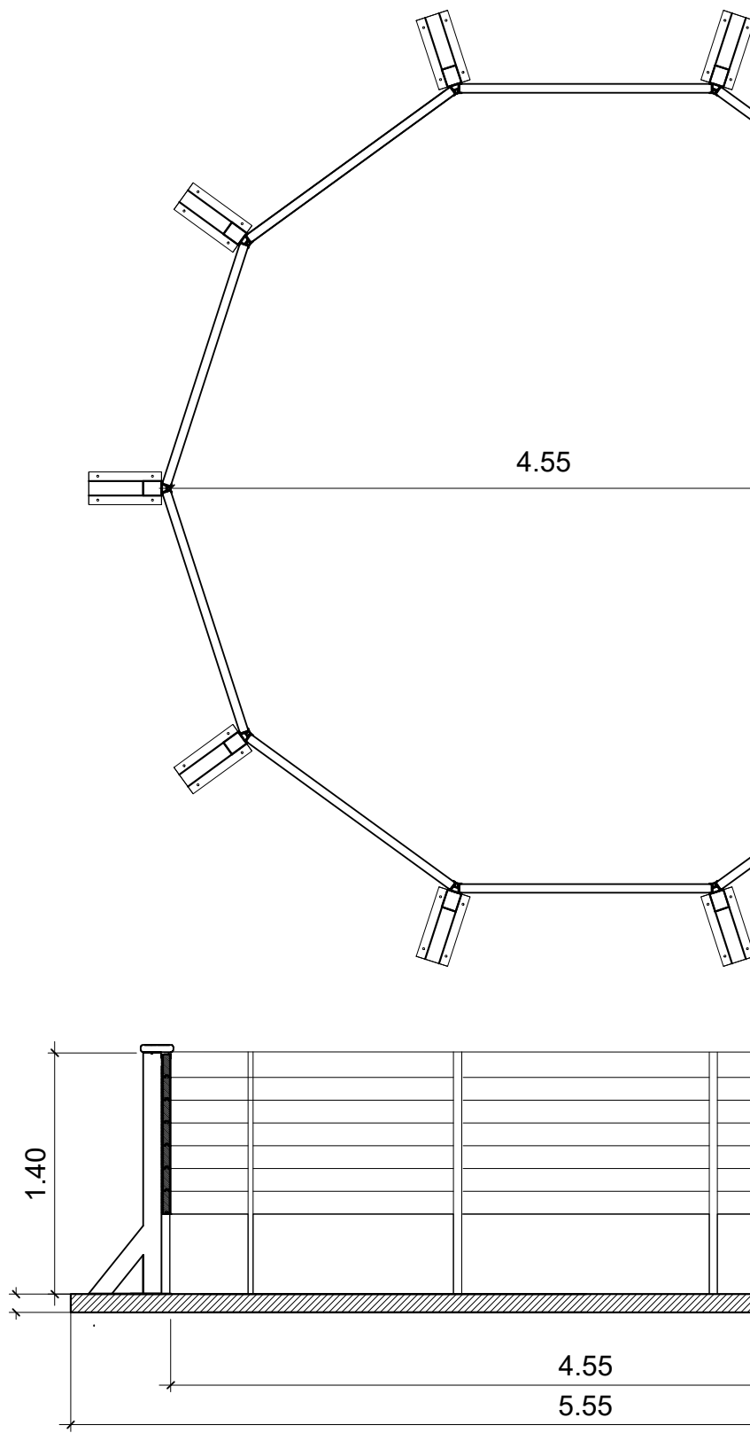
Dalle en béton 0.10m
